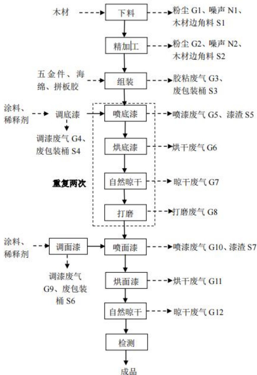
图 3-2 家具生产工艺流程及产污环节图
