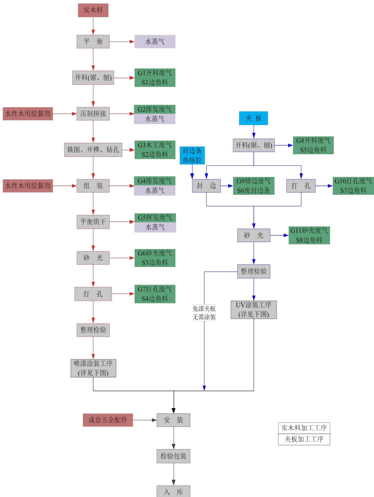
图 3-2 橱柜生产工艺流程及产污环节图
